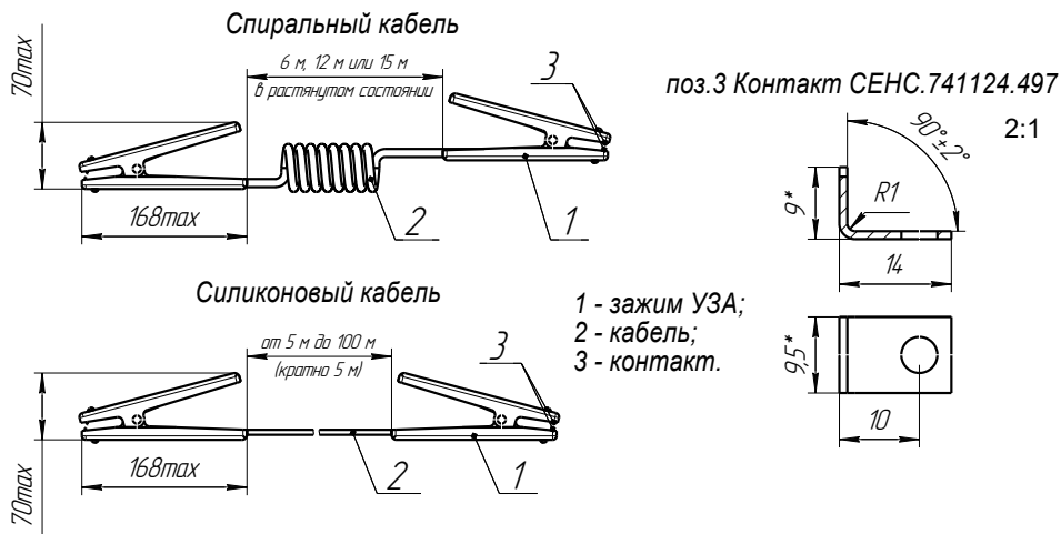
Рисунок 6 – Заземляющий проводник
