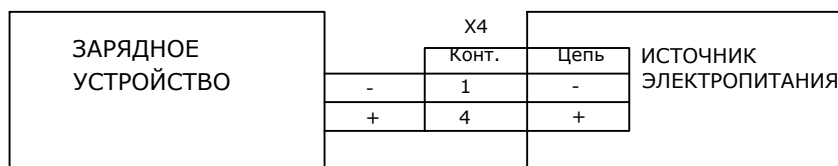
Схема подключения зарядного устройства
